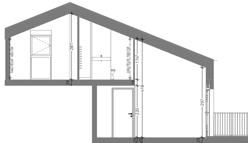
COUPE AA
